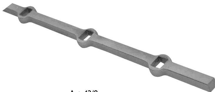
Art. 42/8 ∅ 14 x 14 mm Entre ejes 140 mm agujeros por barra N 14
